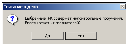
Рис. 8-5. Системное сообщение
