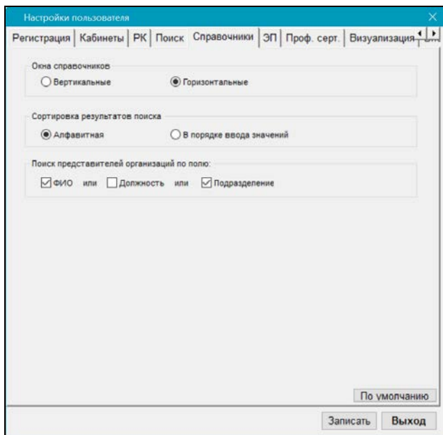
Рис. 22-16. Закладка Справочники
