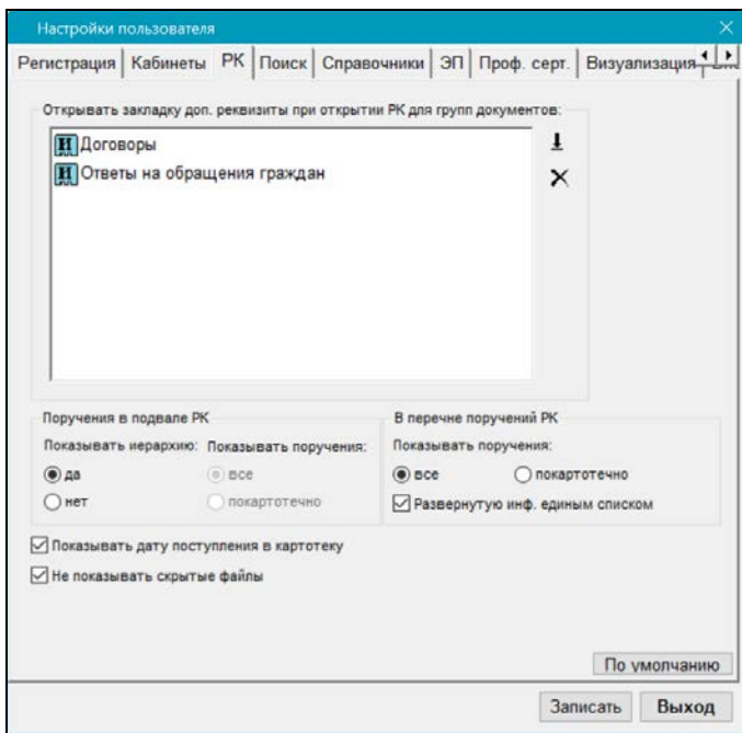
Рис. 22-14. Закладка РК
