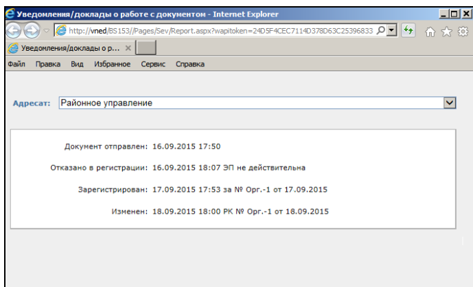
Рис. 20-24. Окно «Уведомления/доклады»
