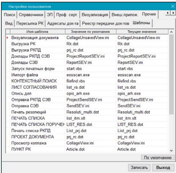
Рис. 22-29. Подзакладка Шаблоны
