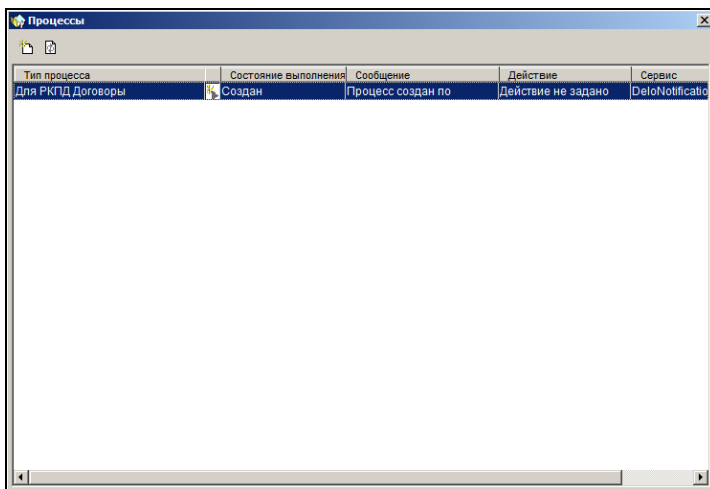
Рис. 2-5. Окно Процессы
