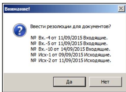
Рис. 10-11. Окно запроса
