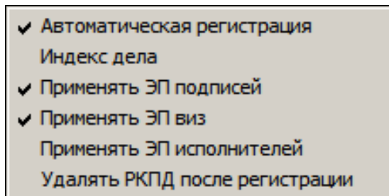
Рис. 13-5. Параметры РКПД
