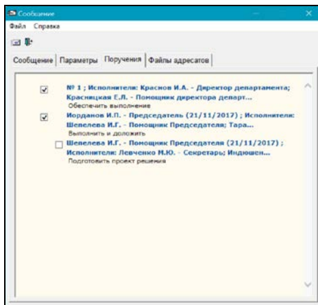
Рис. 20-7 Закладка Поручения
