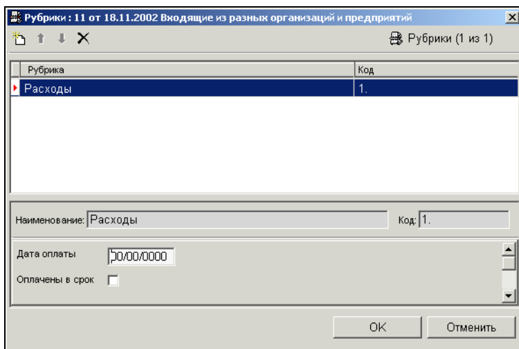
Рис. 5-62. Окно Рубрики
