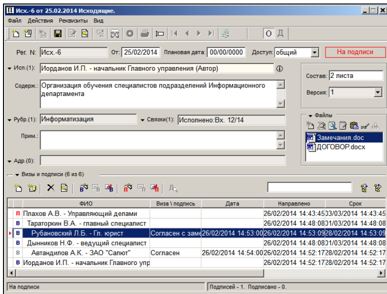
Рис. 13-1. Окно РКПД
