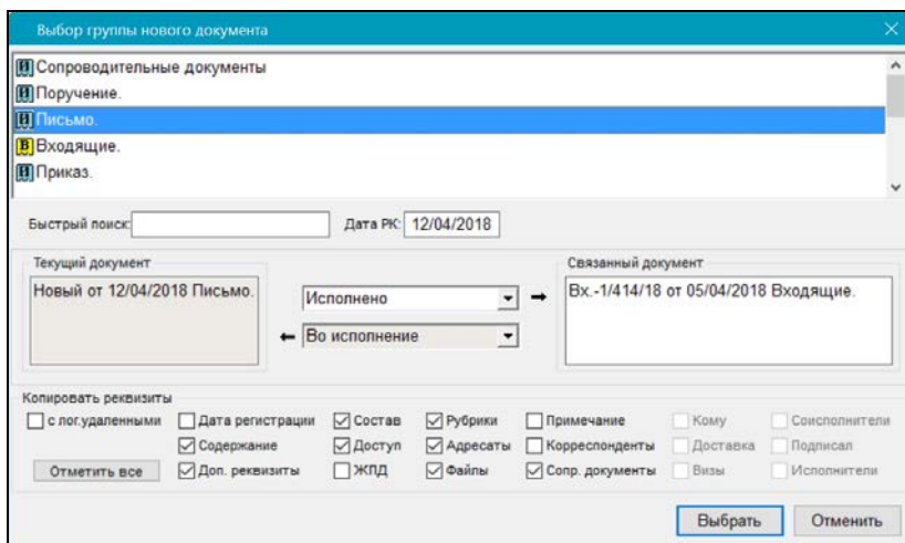
Рис. 5-64. Окно выбора группы нового документа, связанного с исходным документом
