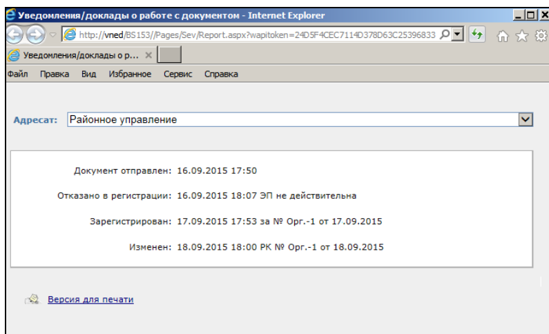
Рис. 18-3. Окно Уведомлений/докладов
