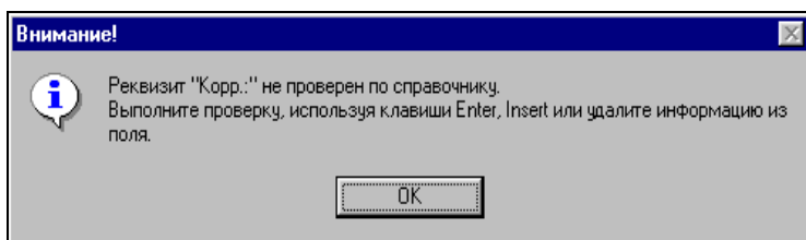
Рис. 5-22. Системное сообщение
