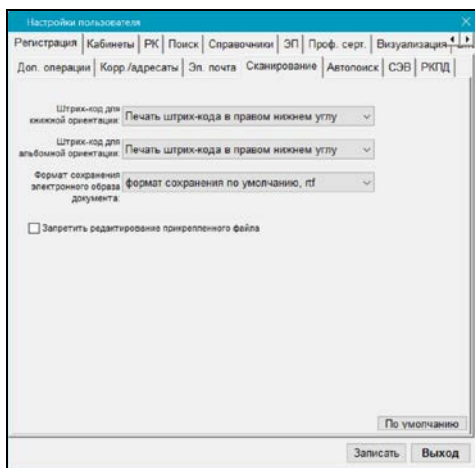
Рис. 22-6. Подзакладка Сканирование
