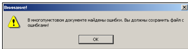
Рис. 10-17. Окно предупреждения
