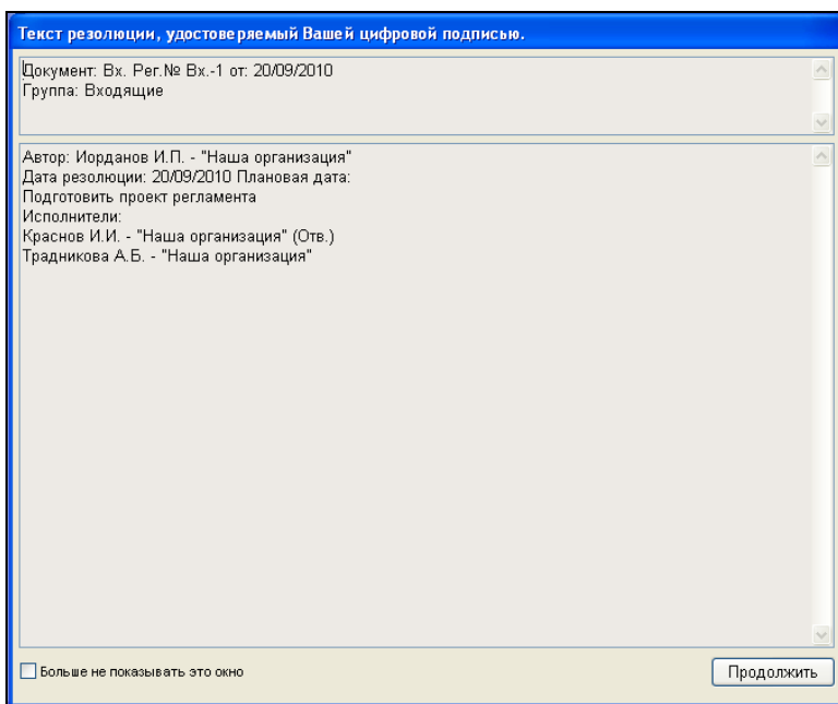
Рис. 10-36. Образ резолюции
