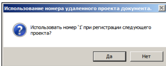
Рис. 13-24. Системное сообщение
