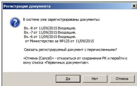
Рис. 5-25. Окно запроса
