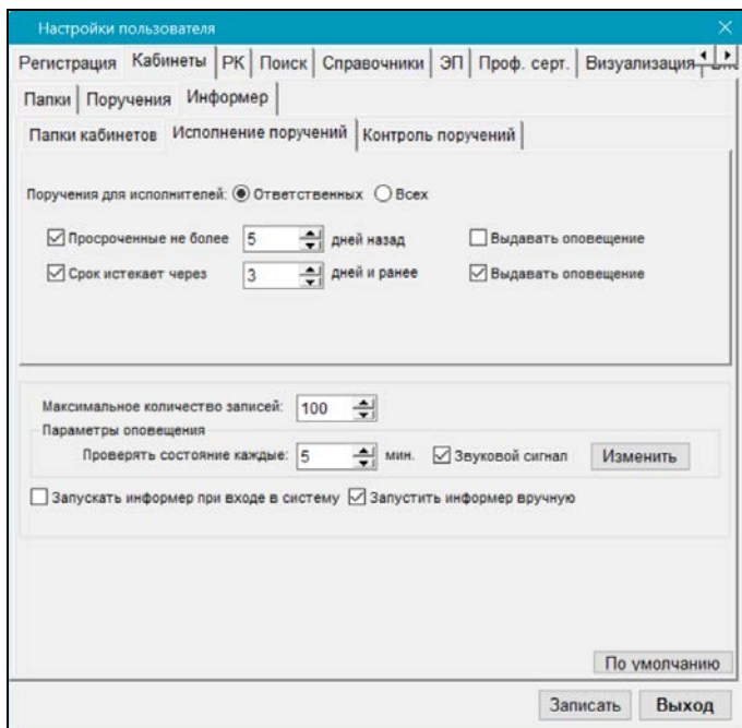
Рис. 22-11. Подзакладка Информер : Исполнение поручений
