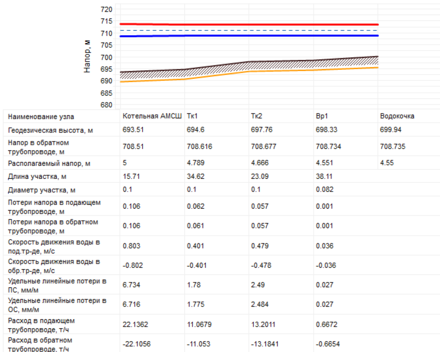
Рисунок 1.3.8.2. Пьезометрический график от котельной «АМСШ» до потребителя «Водокочка»
