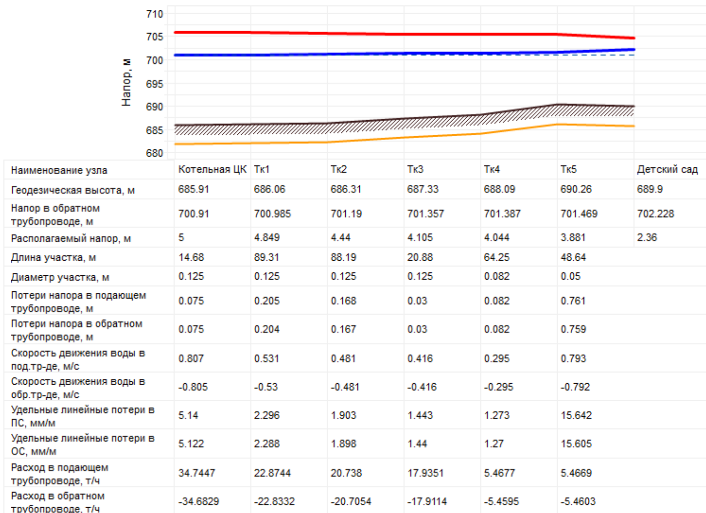
Рисунок 1.3.8.1. Пьезометрический график от Центральной котельной до потребителя «Детский сад»
