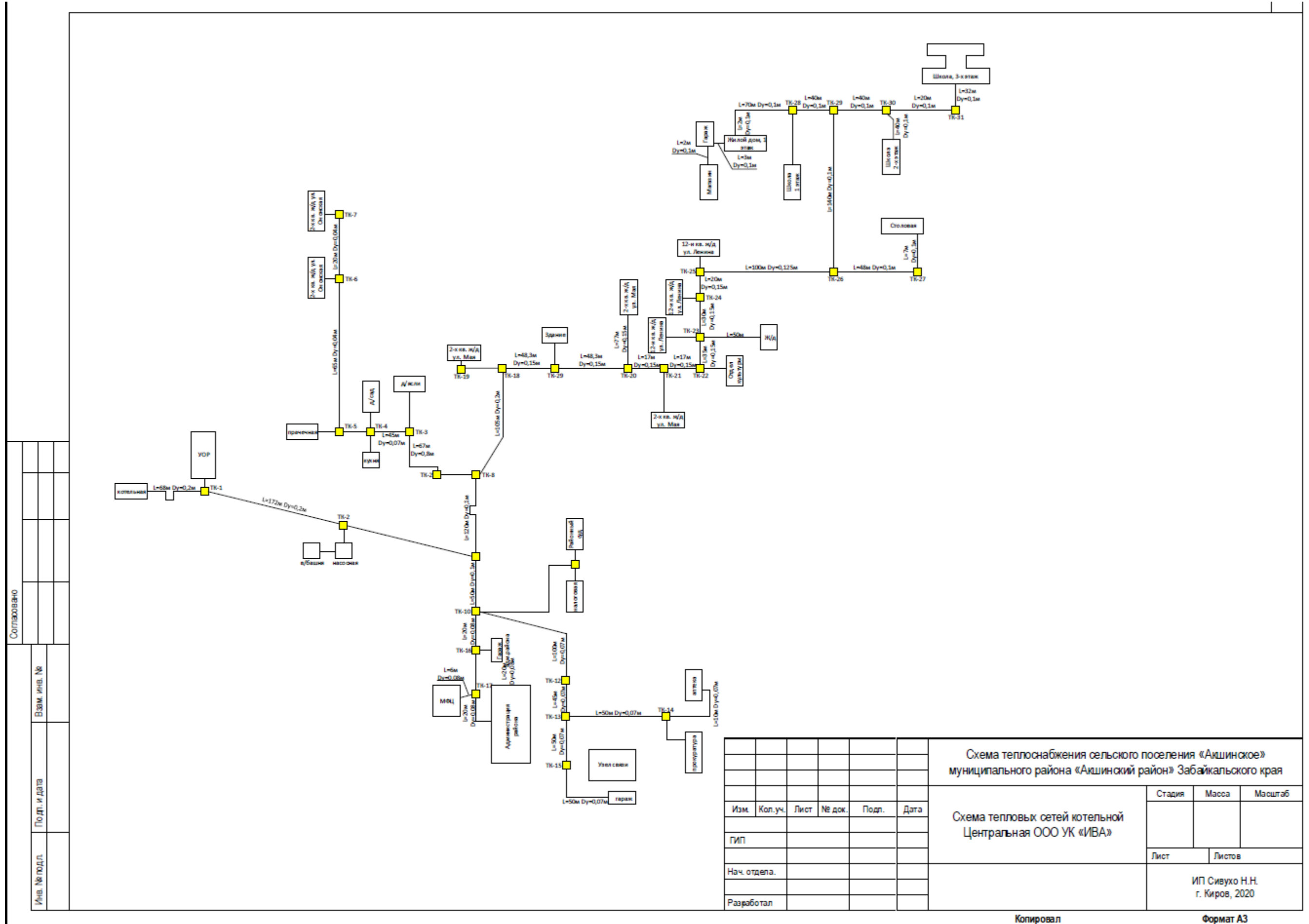
Рисунок 2 - Схема тепловых сетей тепловой сети Центральной котельной
