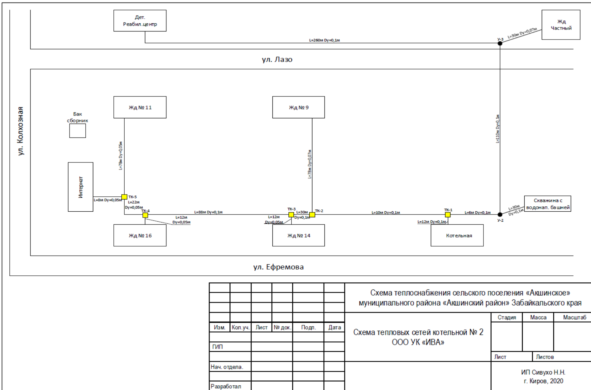
Рисунок 3 - Схема тепловых сетей тепловой сети котельной № 2
