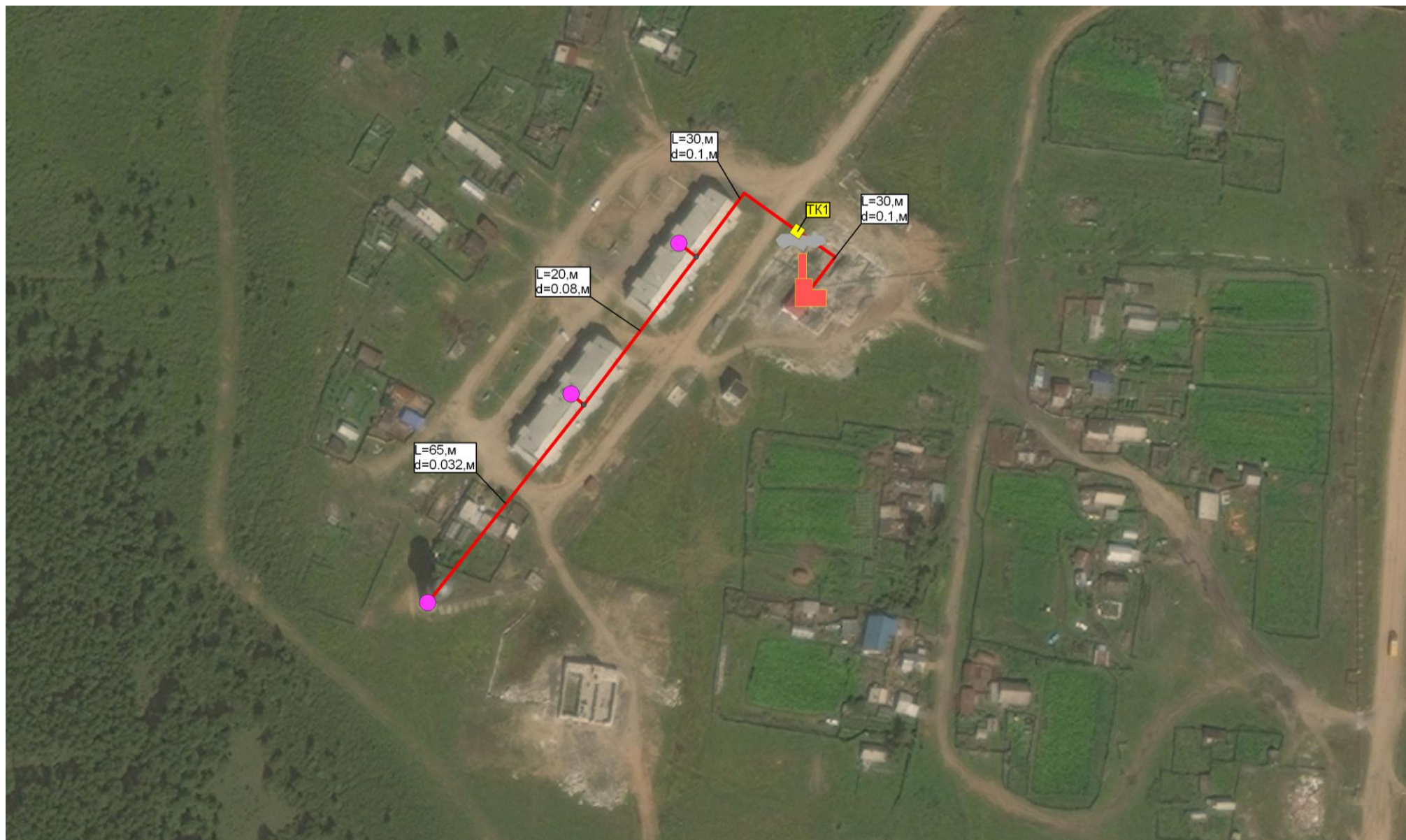
Рис. 2.4 – Схема теплоснабжения муниципального образования сельского поселения "Бушулейское" от котельной №1 на 2014 г.
