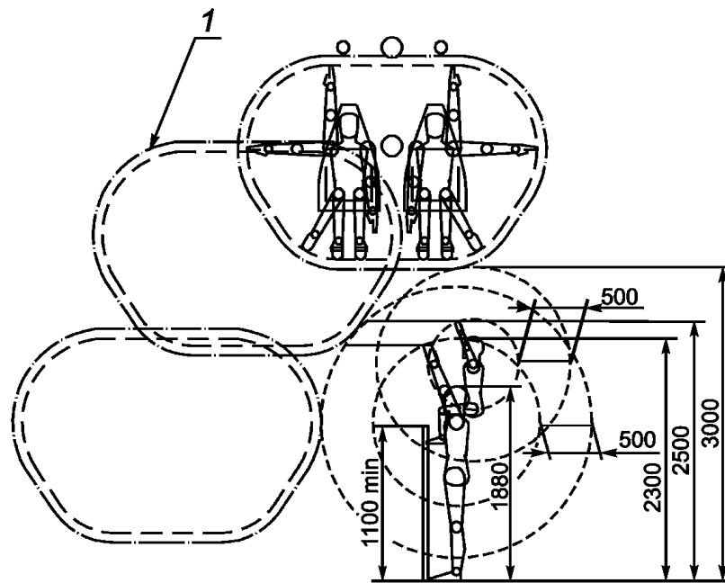
а) Без учета навесов
