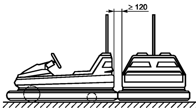
Рисунок 9 - Минимальный зазор для свободно перемещающихся пассажирских модулей
