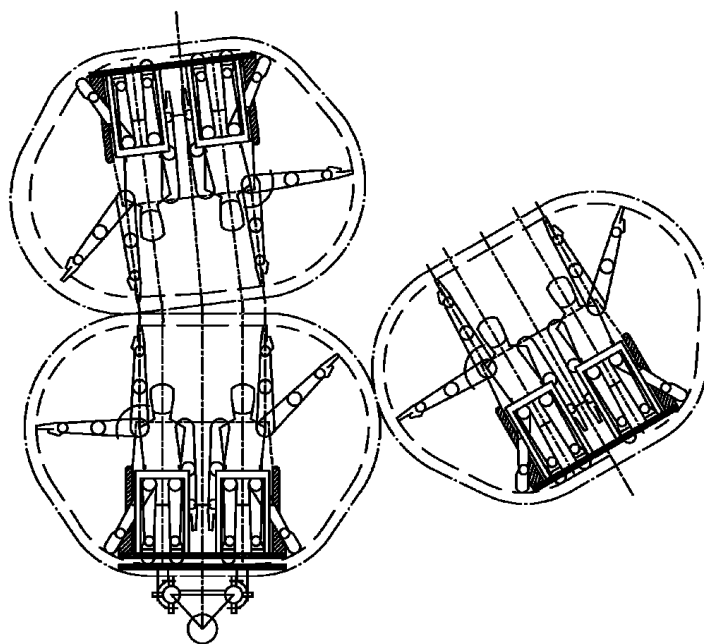
б) Встречное движение
