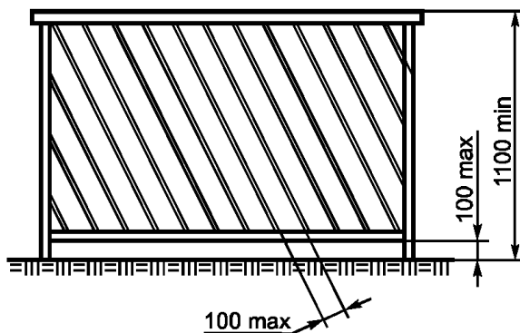
а) Ограждение с наклонным расположением внутренних элементов
