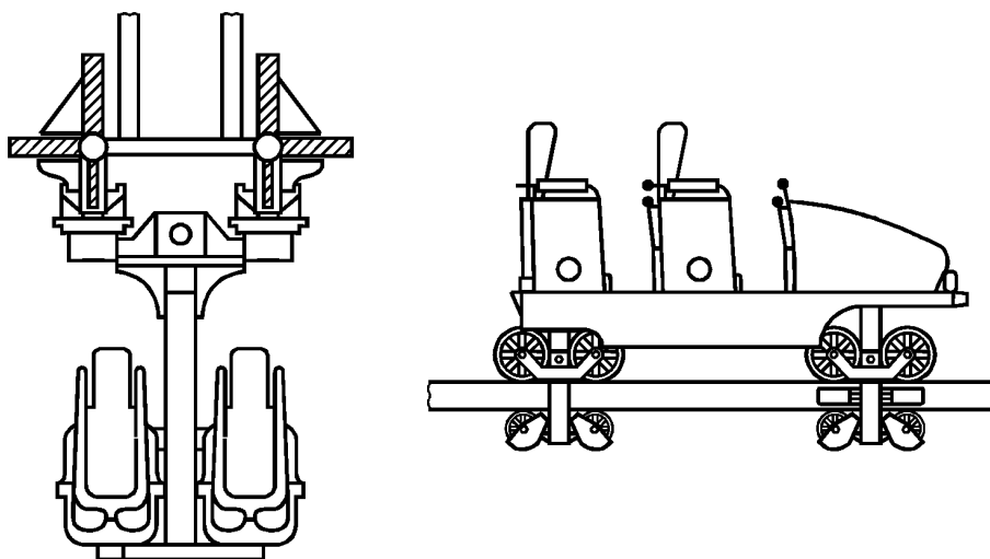
а) Атракцион с направляющими
