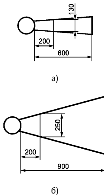
Рисунок 2 - Размеры спиральных и винтовых лестниц
