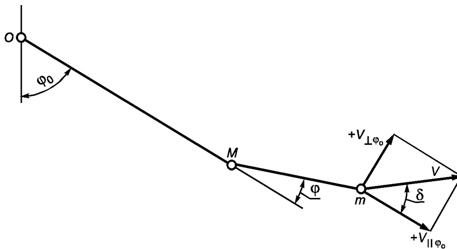
Рисунок B.5. Разложение скорости V
