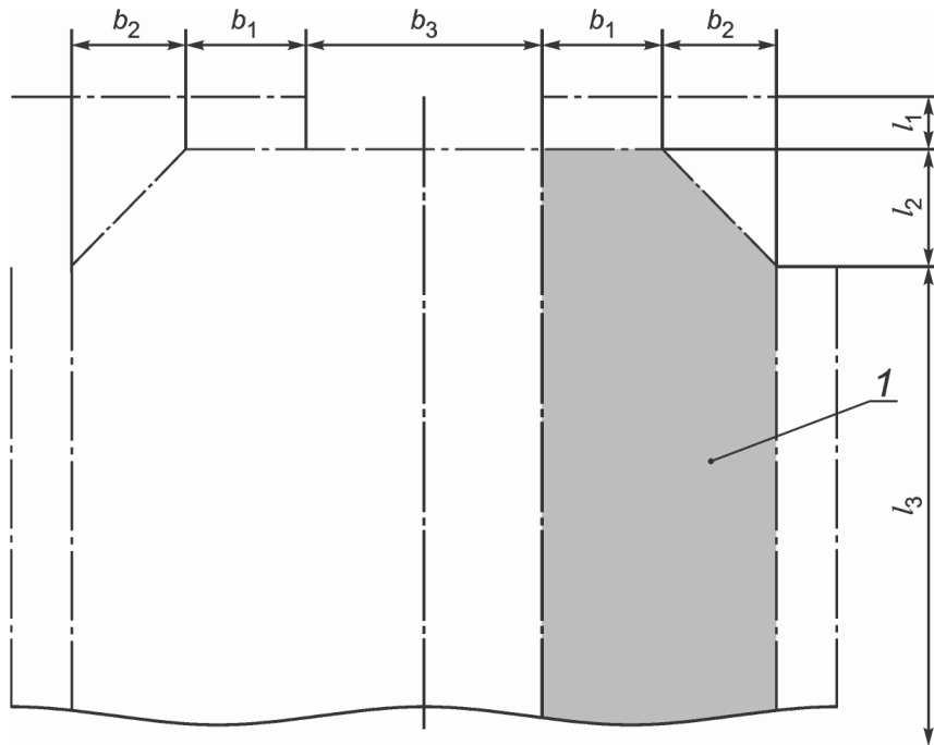
1 - вариант, при котором резервная зона безопасности равна 0 мм (см. 9.3)
