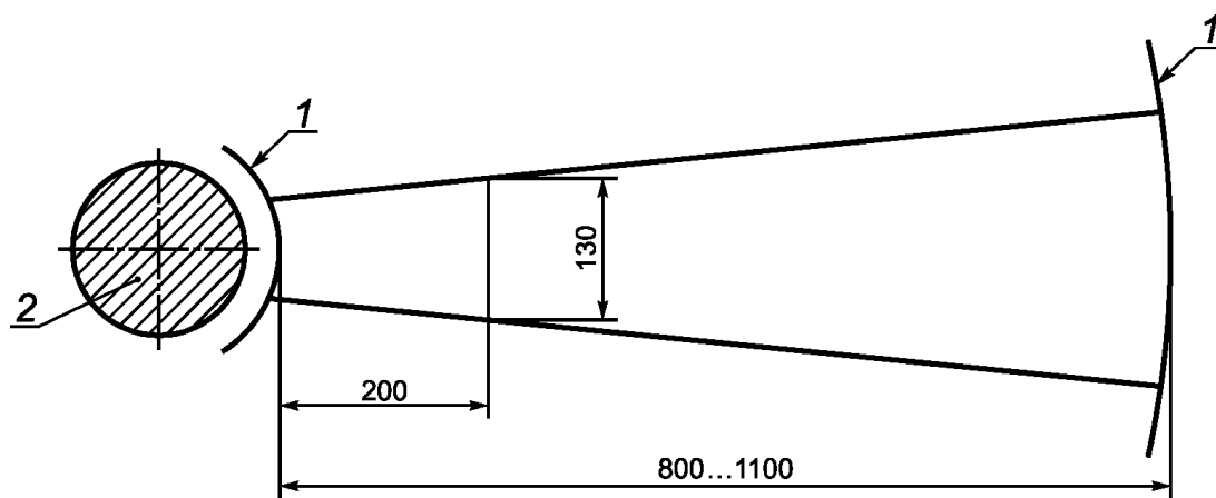
1 - перила; 2 - центральная опора
