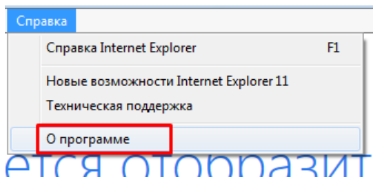
Рисунок 39. О программе
