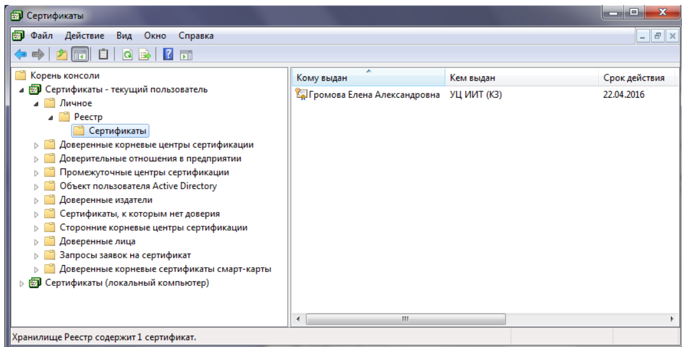
Рисунок 27. Утилита «Сертификаты»
