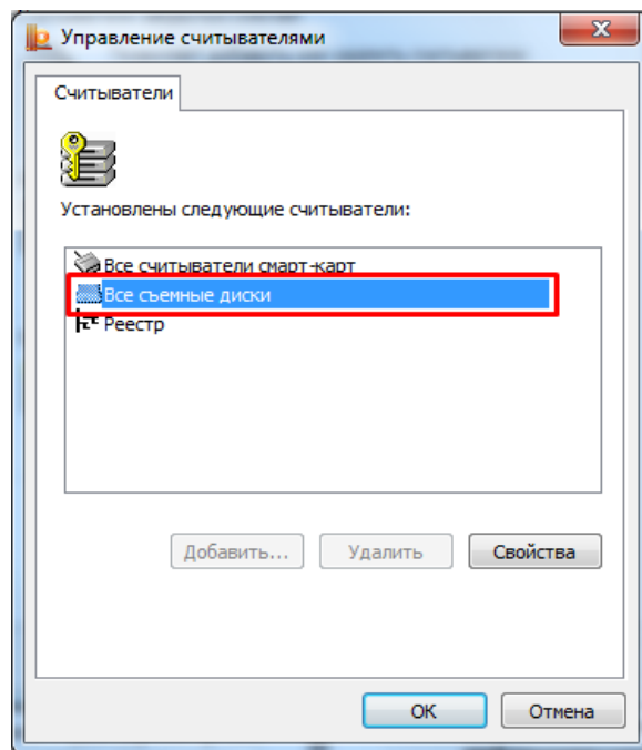
Рисунок 4. Настройка считывателей
