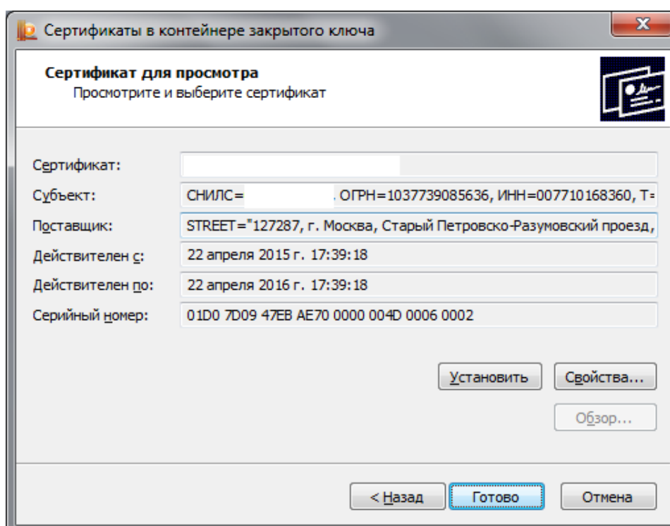
Рисунок 18. Выбор сертификата
