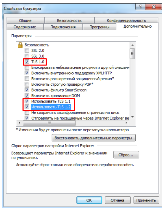
Рисунок 40. Вкладка "Дополнительно"
