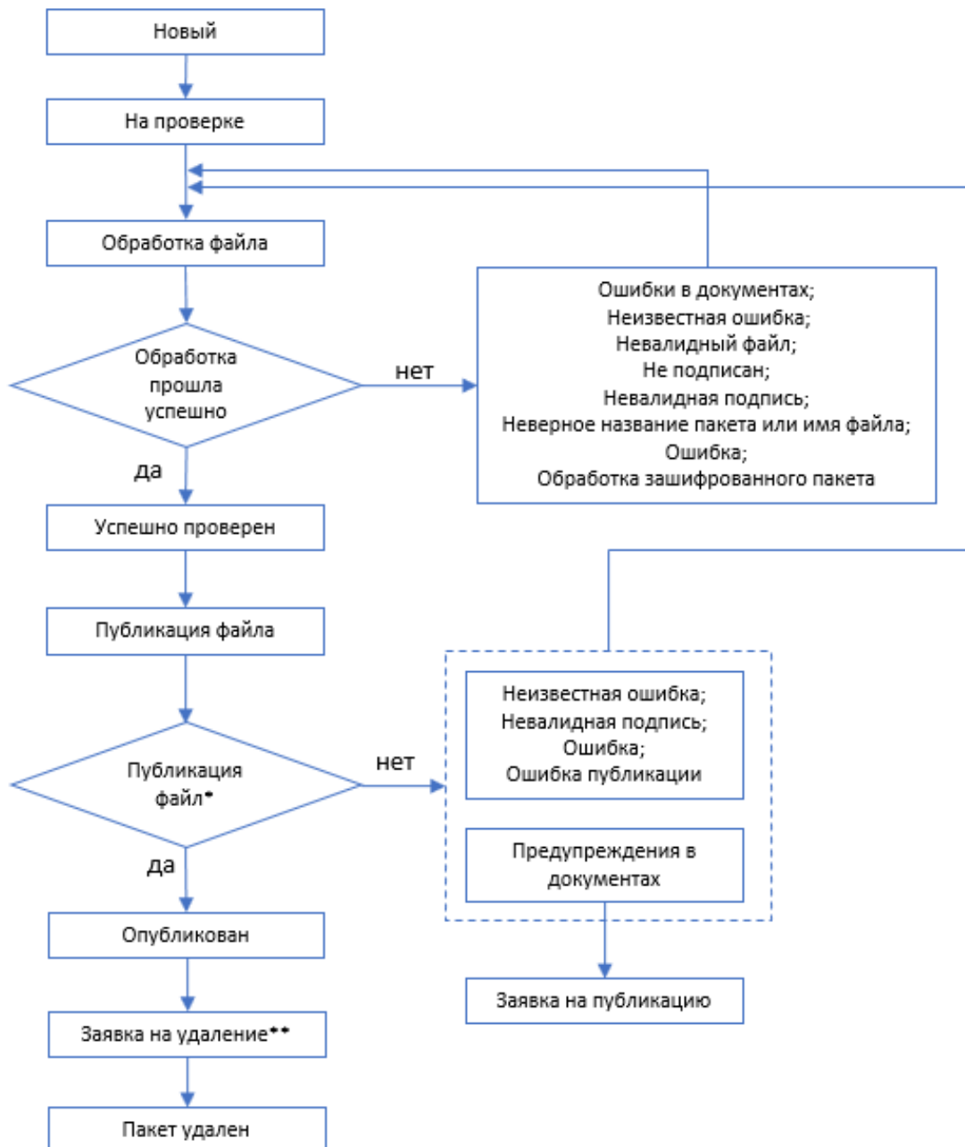
Рисунок 67 – Статусная модель «Пакетов документов»
