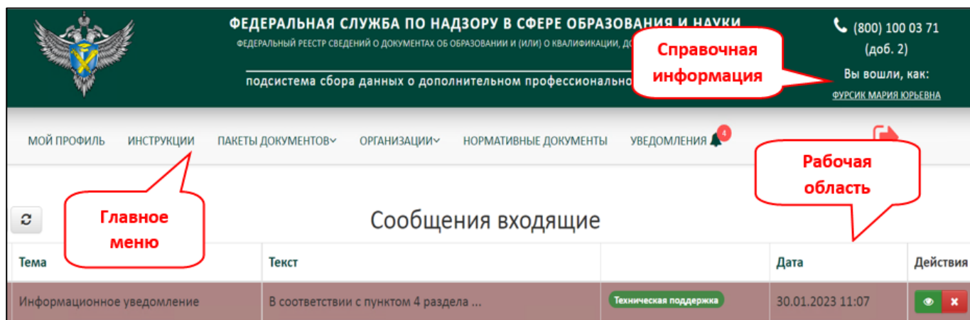
Рисунок 8 – Интерфейс системы
