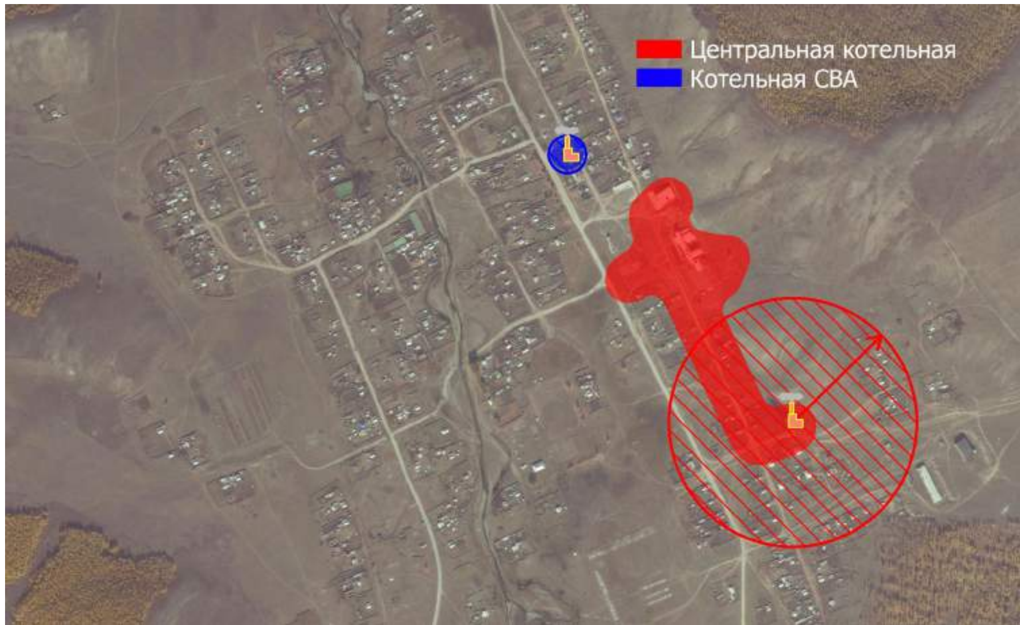
Рис. 5.1 – Радиусы эффективного теплоснабжения с. Догой
