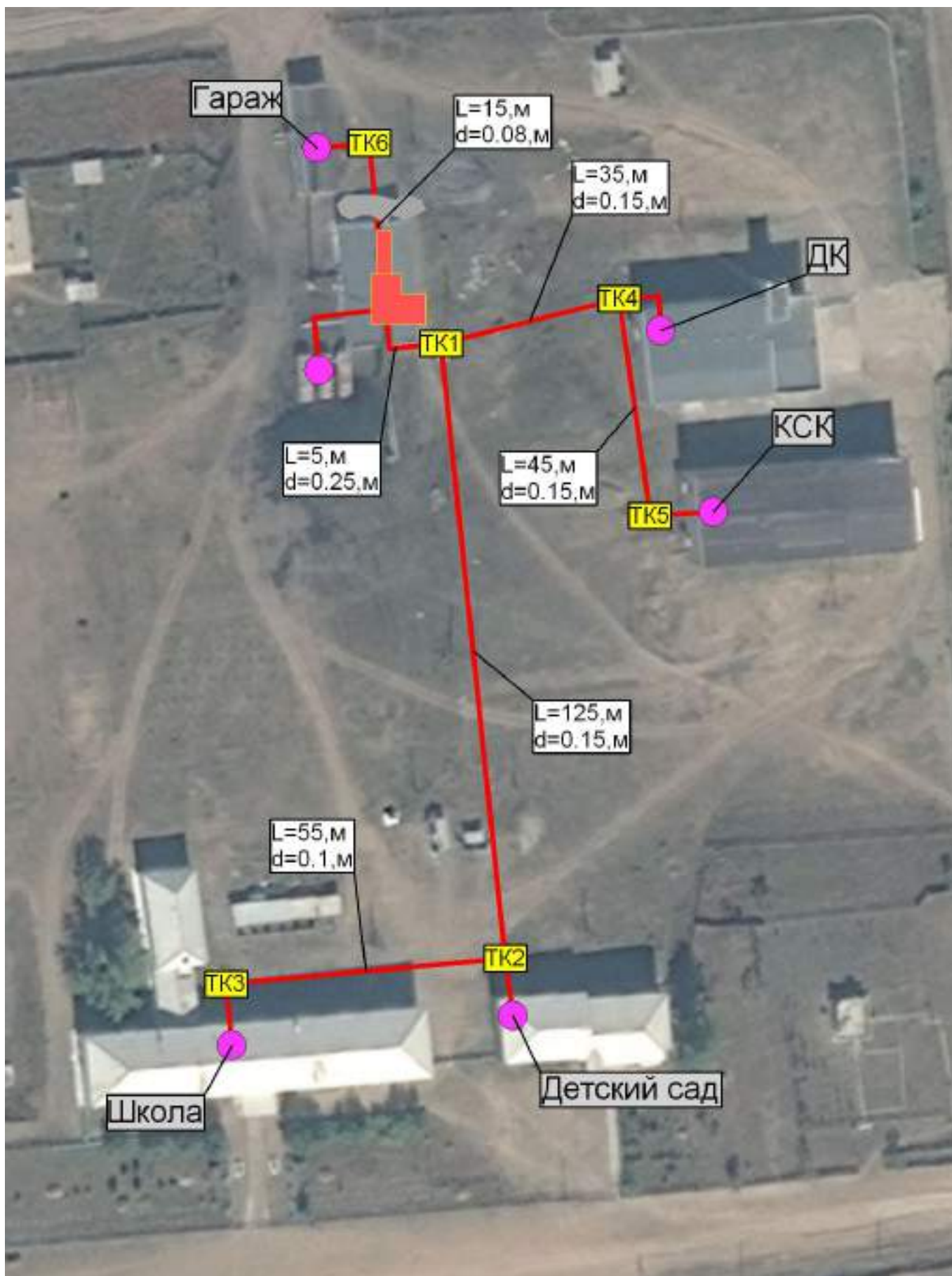
Рис. 2.2 – Схема теплоснабжения муниципального образования сельское поселение "Кусоча" от котельной МОУ КСШ
