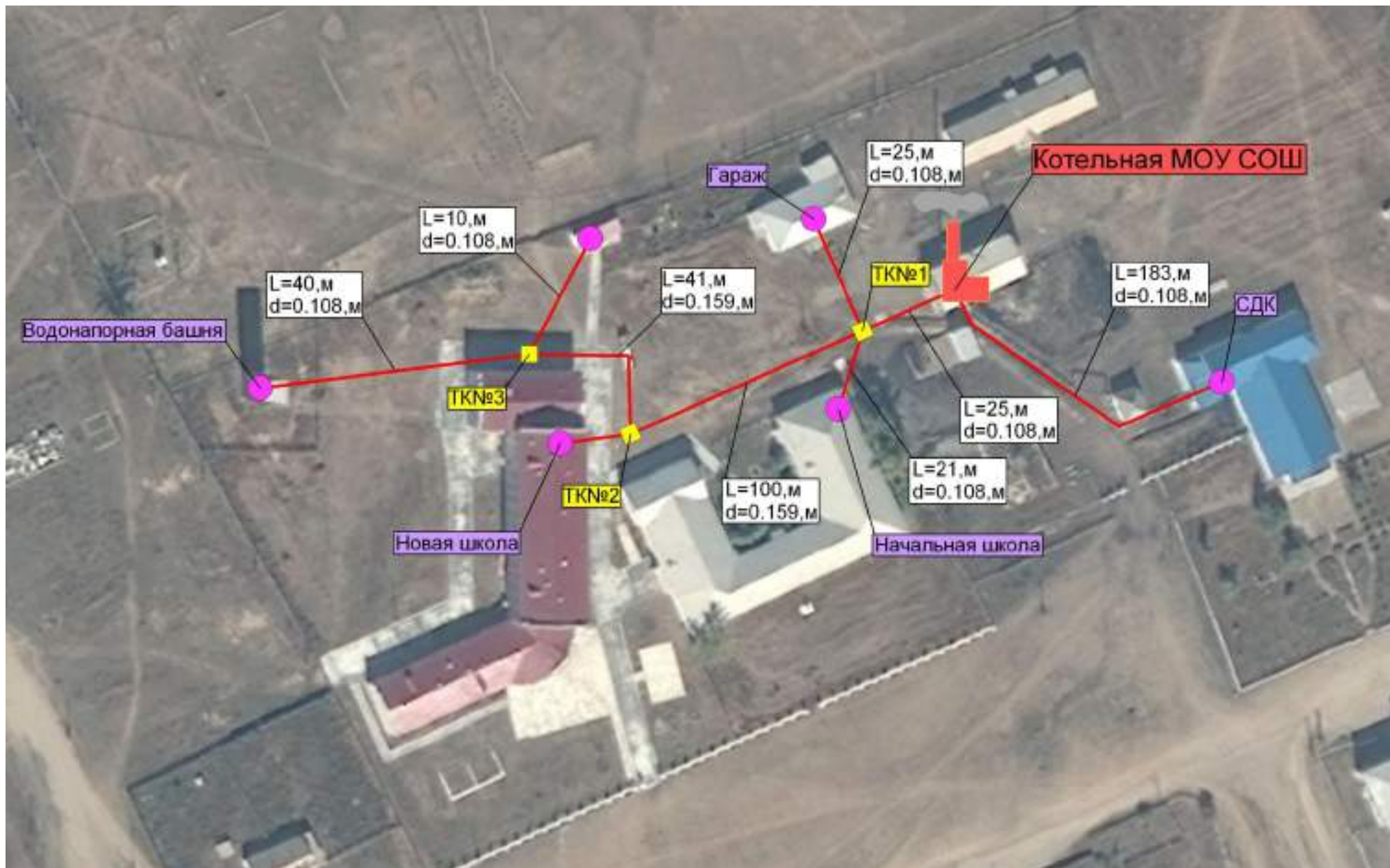
Рис. 2.2 – Схема теплоснабжения муниципального образования сельское поселение «Ортуй» от котельной МОУ СОШ.
