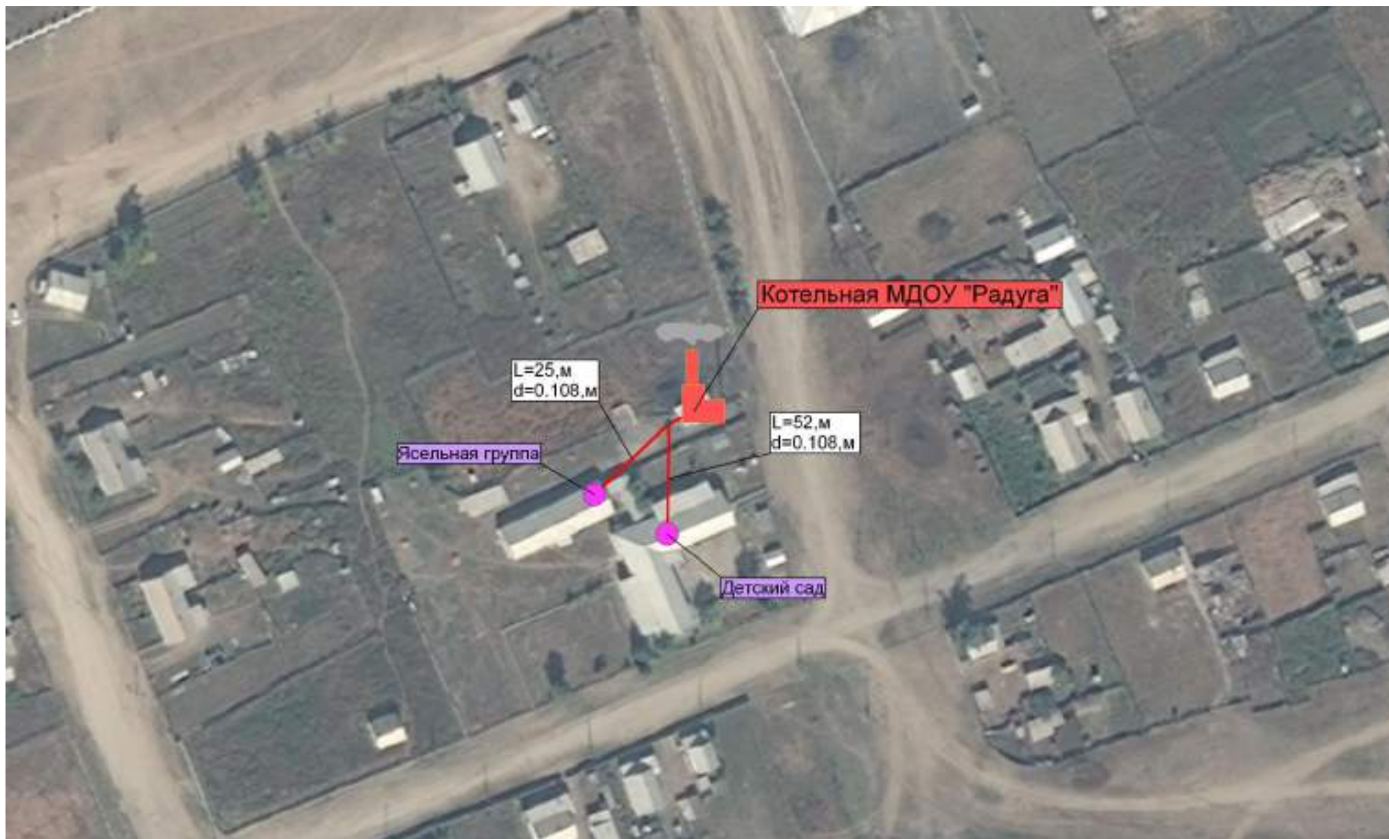
Рис. 2.3 – Схема теплоснабжения муниципального образования сельское поселение «Ортуй» от котельной МДОУ «Радуга»
