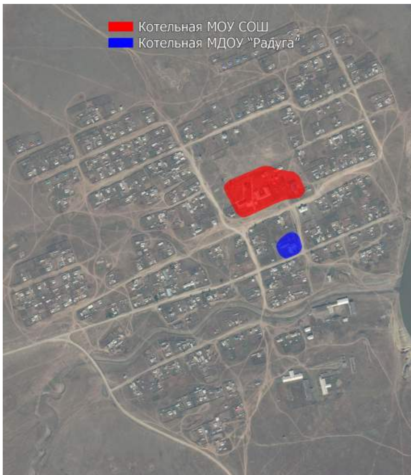
Рис. 2.1 – Зоны действия теплоснабжения муниципального образования сельское поселение «Ортуй».
