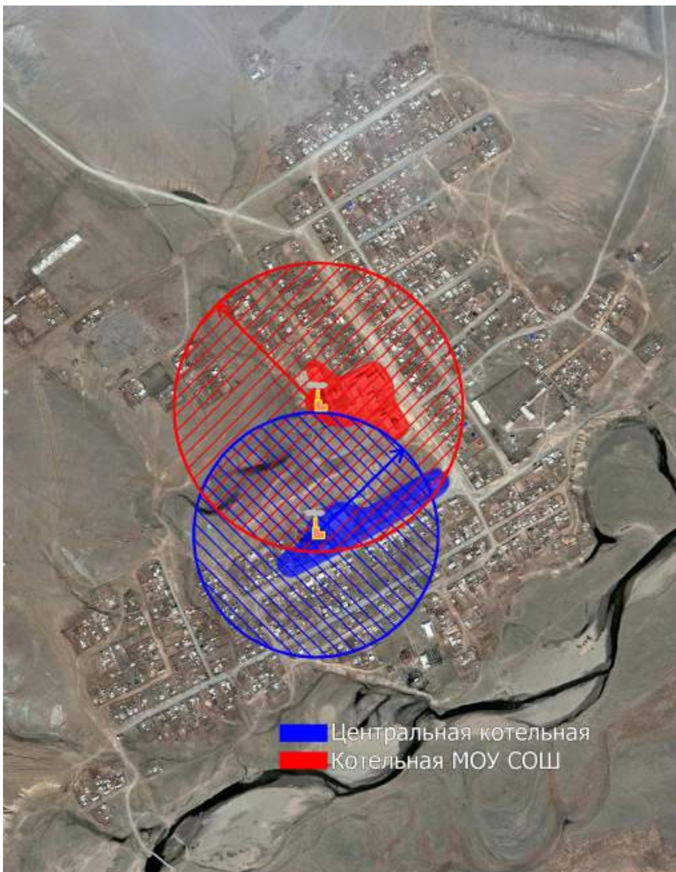
Рис. 5.1 – Радиусы эффективного теплоснабжения с. Цаган-Ола
