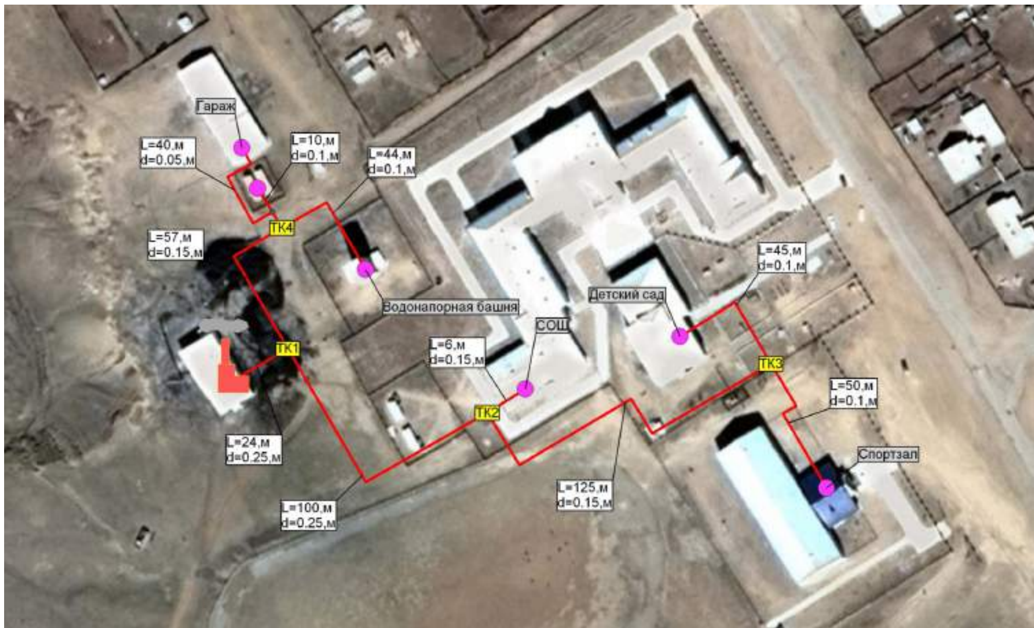
Рис. 2.3 – Схема теплоснабжения муниципального образования сельское поселение "Цаган-Ола" от котельной МОУ СОШ
