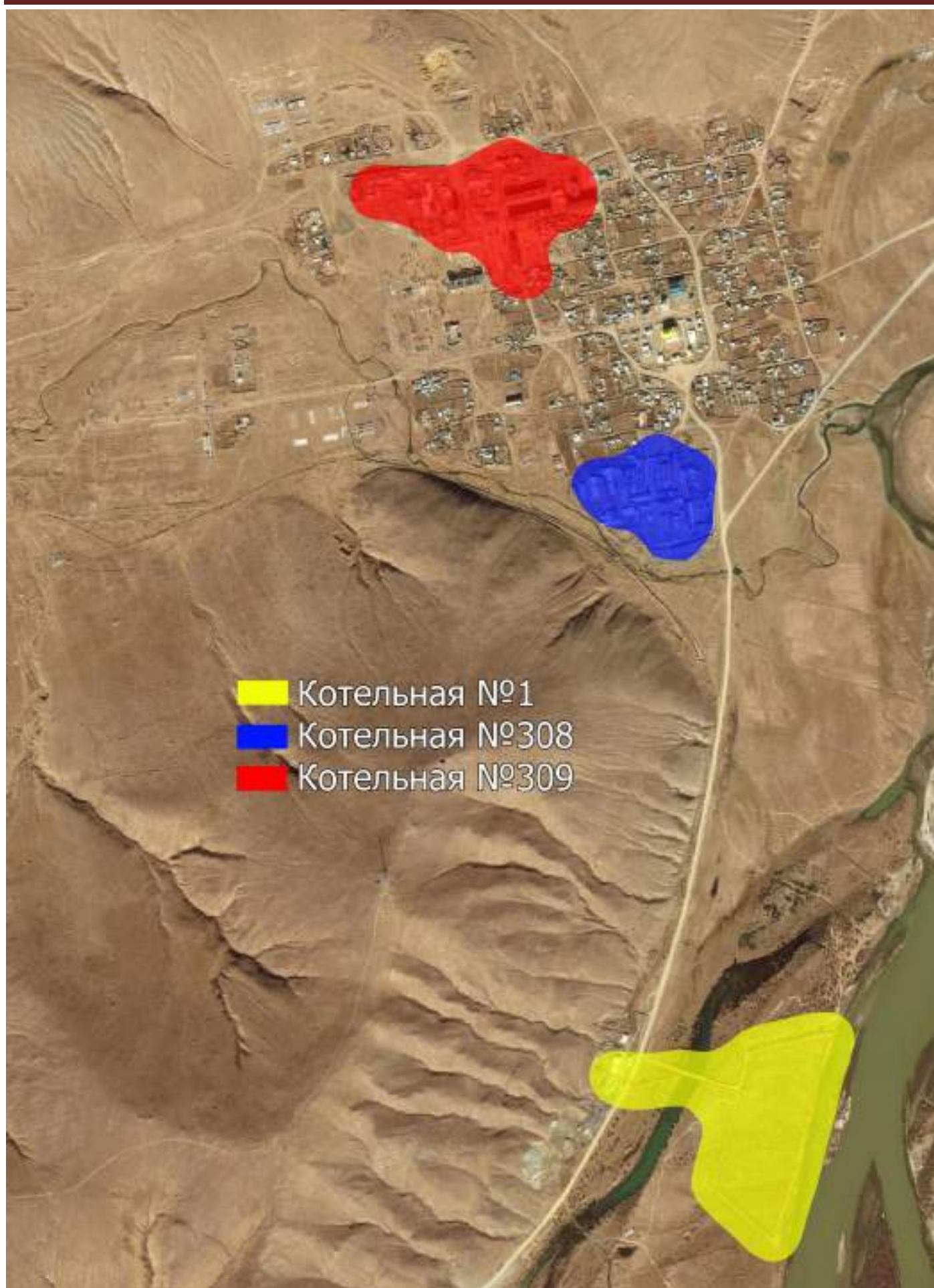
Рис. 2.1 – Зоны действия систем теплоснабжения села Цугол
