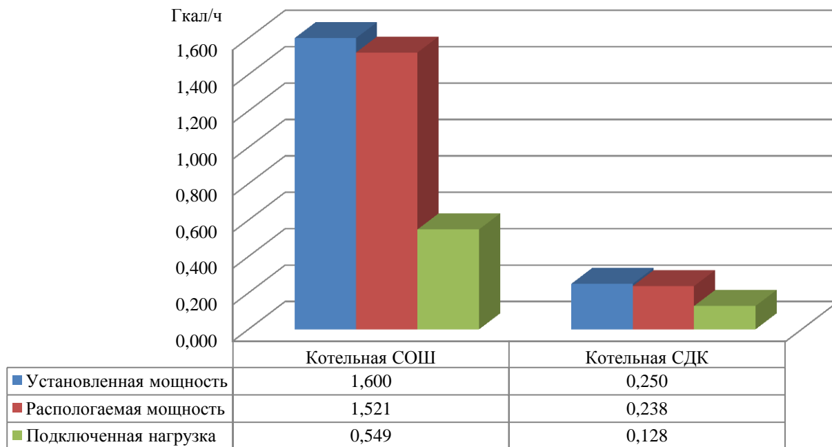
Рис. 2.1 – Загрузка котлоагрегатов котельных
