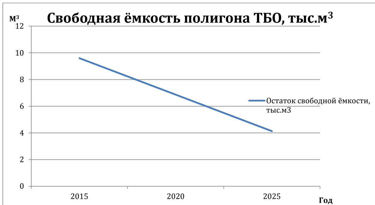
Рис. 3.5.1. – График уменьшения ёмкости полигона ТБО
