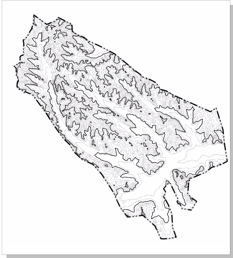
ИЗОЛИНИИ РЕЛЬЕФА
