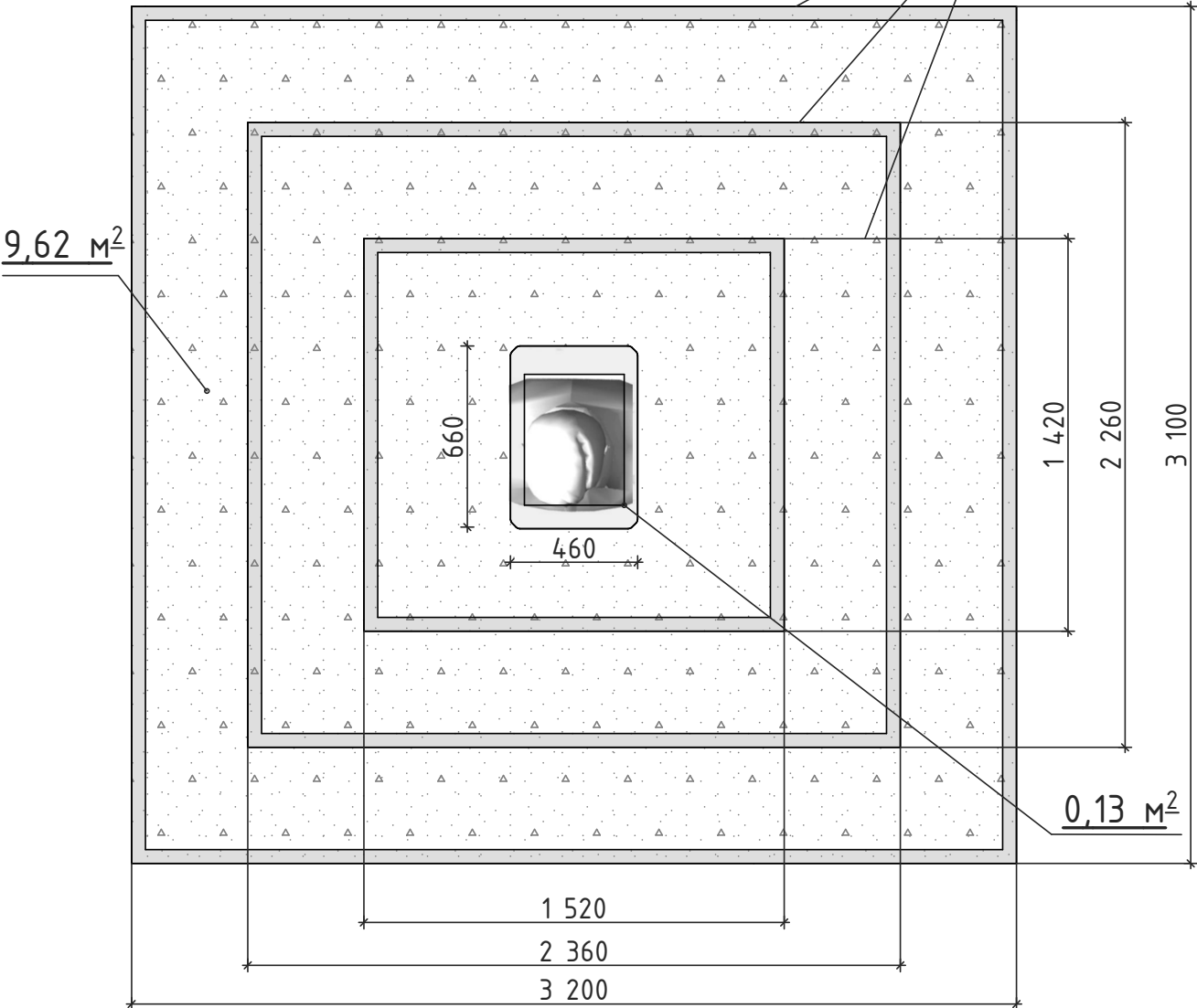
План бюста В.И. Ленину с пьедесталом и ступенями
