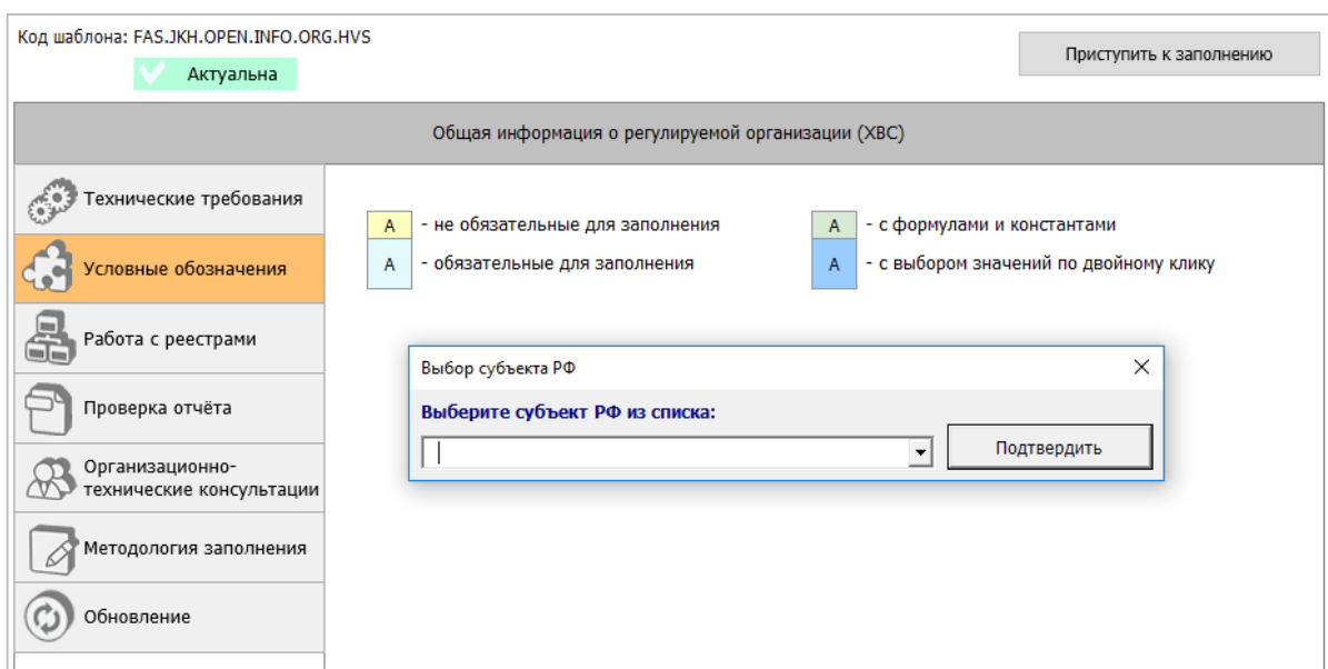
Рисунок 2 - Лист «Инструкция»
